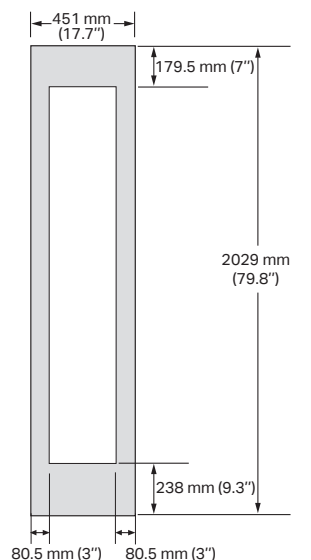
COLONNA DA INCASSO DA 457 mm (18")
